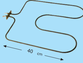
CR 114 325 Fırın Boru Rezistanı 220V. 1200W. (6.5 Ø-Cr-ni)
