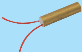
CR 113 125 Pano Fişek Rezistanslar 220V.-100W Boy:65 mm Çap:16mm
