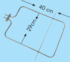
CR 114 341 Fırın Boru Rezistanı 220V. 1200W. (6.5Ø-Cr-ni)
