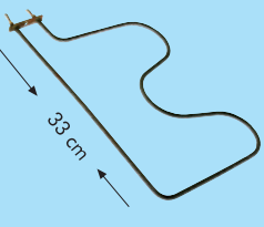
CR 114 335 Fırın Boru Rezistanı 230V. 650W. (6.5Ø-Cr-ni)
