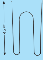
CR 114 295 (M) Tipi Fırın Boru Rez. (KUMTEL) 220V.1000W. (6.5 Ø-Cr-ni)
