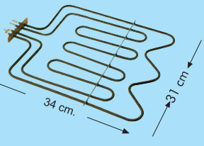
CR 114 354 Fırın Boru Rezistanı 220V. 3500W. (6.5 Ø-Cr-ni)
