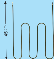
CR 114 305 Fırın Boru Rezistanı 220V. 1000W. (6.5 Ø-Cr-ni)
