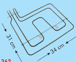
CR 114 362 Arçelik Fırın Rezistanı 220V. 2200W. (6.5 Ø-Cr-ni)
