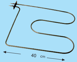
CR 114 329 Fırın Boru Rezistanı 220V. 750W. (6.5 Ø-Cr-ni)
