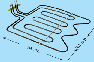
CR 114 356 Fırın Boru Rezistanı 220V. 3500W. (6.5 Ø-Cr-ni)
