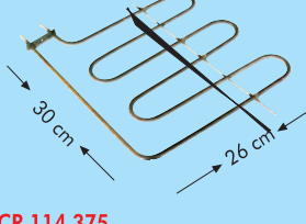
CR 114 375 Mini Arçelik Fırın Boru Rez. 220V. 2000W. (6.5 Ø-Cr-ni)
