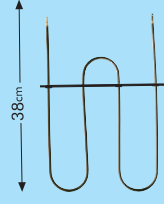
CR 114 293 (M) Tipi Fırın Boru Rezistanı 220V.1000W. (6.5 Ø-Cr-ni)
