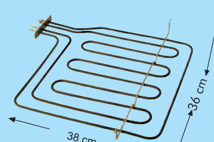
CR 114 358 Fırın Boru Rezistanı 220V. 3500W. (6.5 Ø-Cr-ni)
