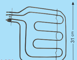
CR 114 359 Küçük Fırın Boru Rezistanı 230V. 3000W. (6.5 Ø-Cr-ni)
