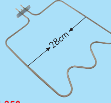
CR 114 350 Küçük Fırın Boru Rezistanı 220V. 1200W. (6.5Ø-Cr-ni)
