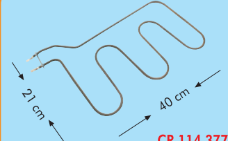
CR 114 377 Arçelik Fırın Rezistanı 220V. 1500W. (6.5 Ø-Cr-ni)
