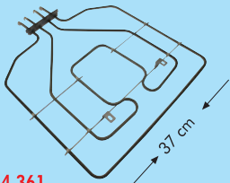
CR 114 361 Arçelik Fırın Rezistanı 220V. 2800W. (6.5 Ø-Cr-ni)
